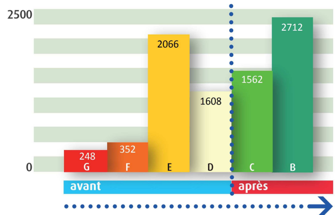
Classes énergétique avant et après travaux
