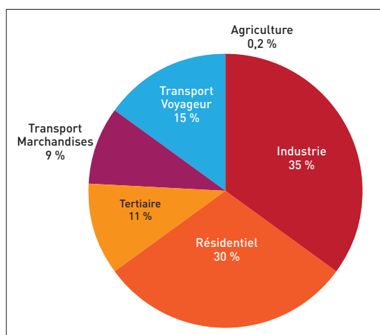
Figure 93 : Scénario «Objectifs Grenelle» 2020 : Contribution des différents secteurs à la baisse des consommations énergétiques, Energies Demain 2011
