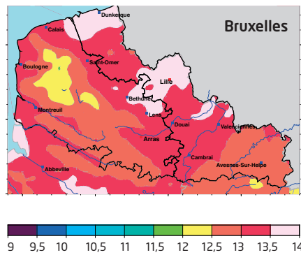
Figure 41 : Moyenne annuelle des températures en région Nord-Pas de Calais (en °C) : aujourd'hui, à l'horizon 2050 et à l'horizon 2080, selon les scénarios B1 (à gauche) et B2 (à droite) (Météo-France - 2011)
