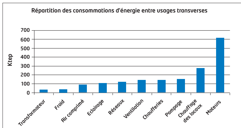
Figure 83 : Répartition des consommations des usages transverses dans le secteur industriel en Nord-Pas de Calais (E&E Consultant - 2005)
