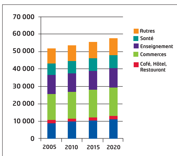
Figure 75 : Hypothèses de croissance du parc tertiaire en milliers de m² (Energies Demain - 2011)
