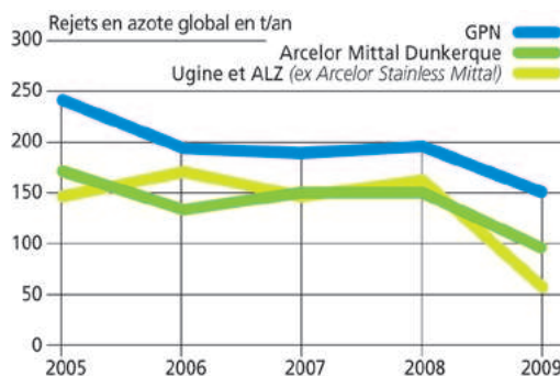
Les principaux rejets industriels en azote global (supérieurs à 50 t/an) et leur évolution
