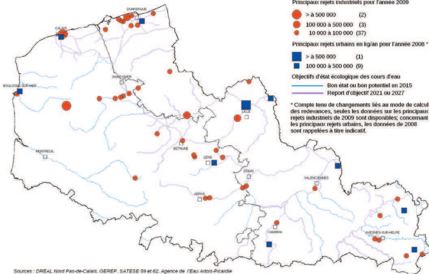
La répartition des principaux rejets industriels et urbains de MES en 2009
