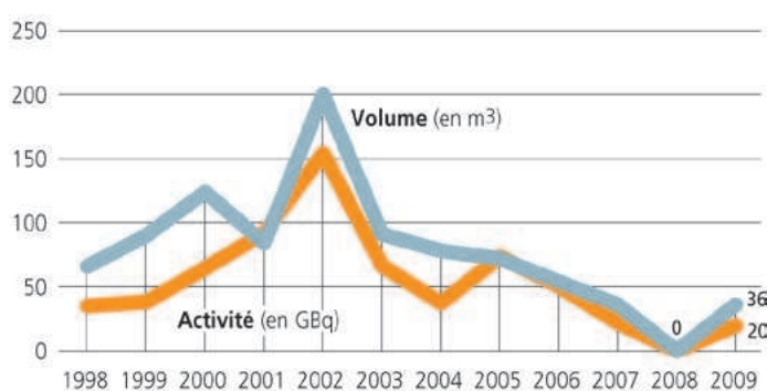
Évolution du volume et de l'activité des effluents actifs enlevés à la Somanu
