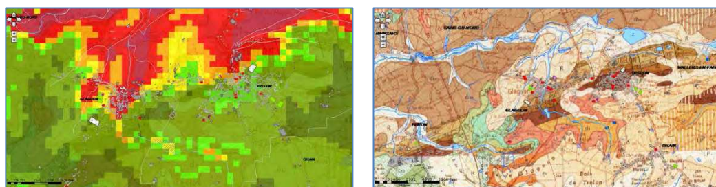
Secteur de Glageon (Ruisseau de Pont de Sains et de Lorrain Fossé), en domaine paléozoïque
