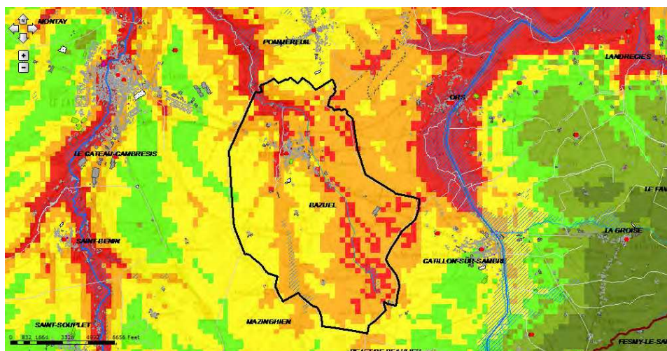
Le secteur de Bazuel
