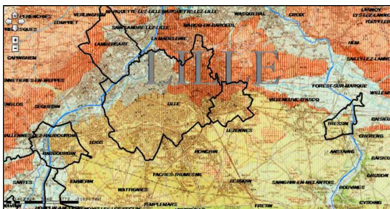
Géologie du secteur de Lille (Craie très proche du sol, recouverte de Tertiaire)
