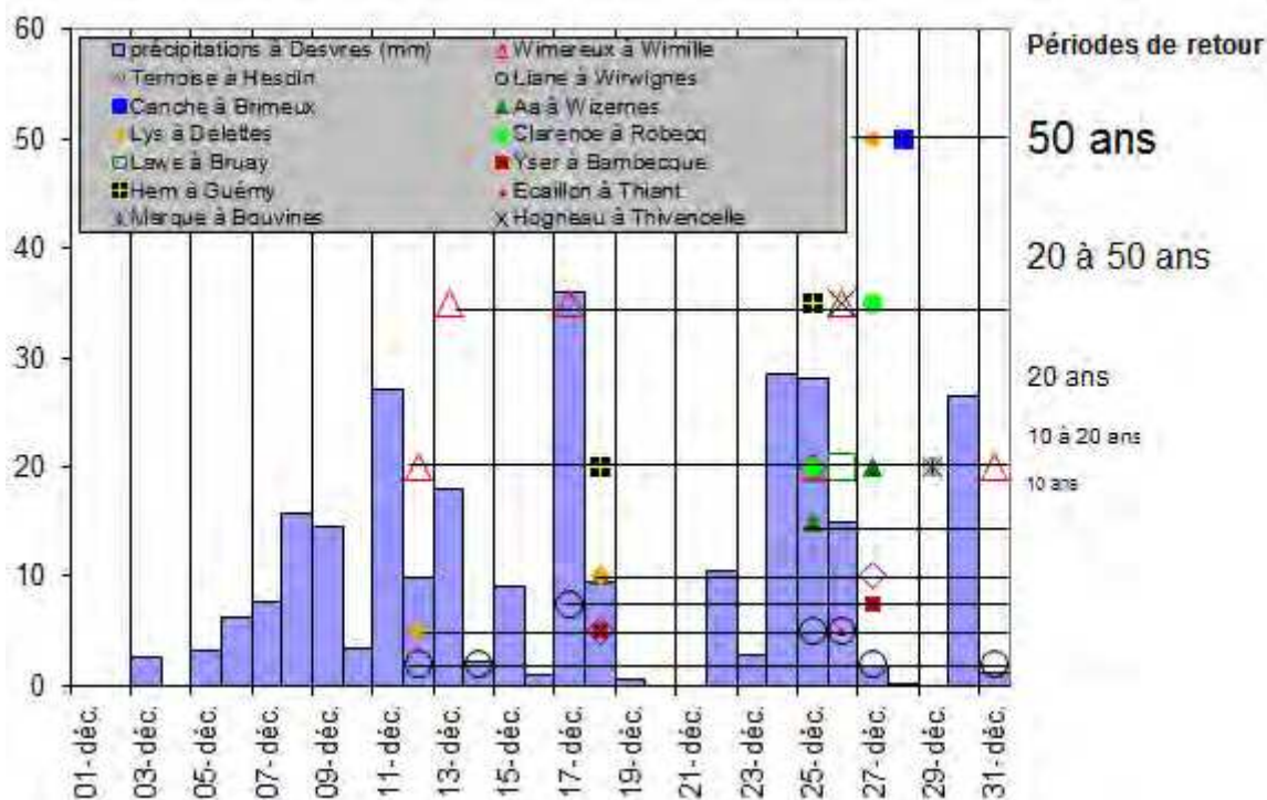
Figure 7 : Précipitations relevées à Desvres et périodes de retour des crues des différents cours d'eau. Le graphique a été reconstitué par le CEMAGREF, à partir des données brutes issues du document. [Source : Rapport des crues du mois de décembre 1999]
