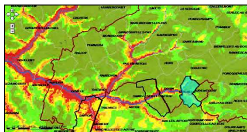
Coigneux et Saint Léger sur Authie, sur l'Authie (Somme)
