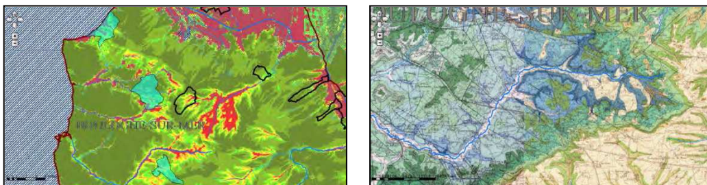
La boutonnière du Boulonnais (à g. la sensibilité, à dr. les terrains jurassiques et la haute vallée de la Liane)
