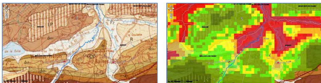
Secteur de Trélon, Wallers et Baives (Helpe Majeure et ruisseau de Baive), en domaine paléozoïque
