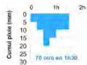
Figure 19 : Cumul de pluie approximé du 7 juin 2007 sur 1 h 30 sur le secteur d'Estreux, par pas de temps de 15 minutes, d'après les images radar. [Source : Thèse J. DOUVINET]
