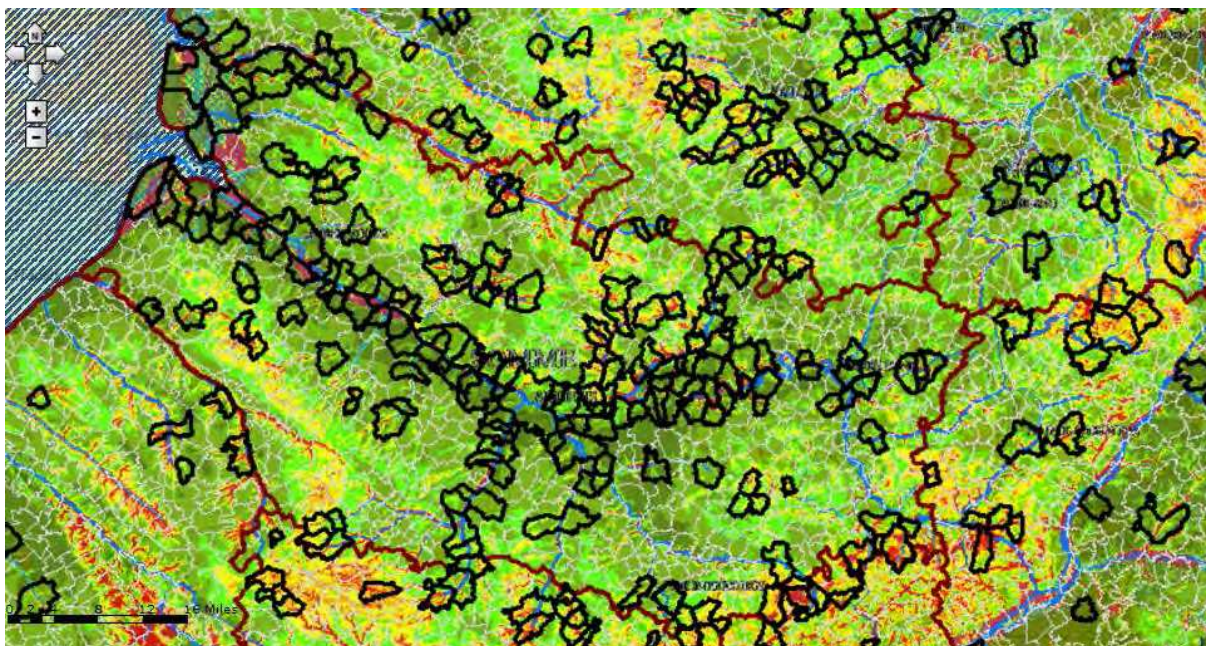
Sensibilité du département de la Somme
