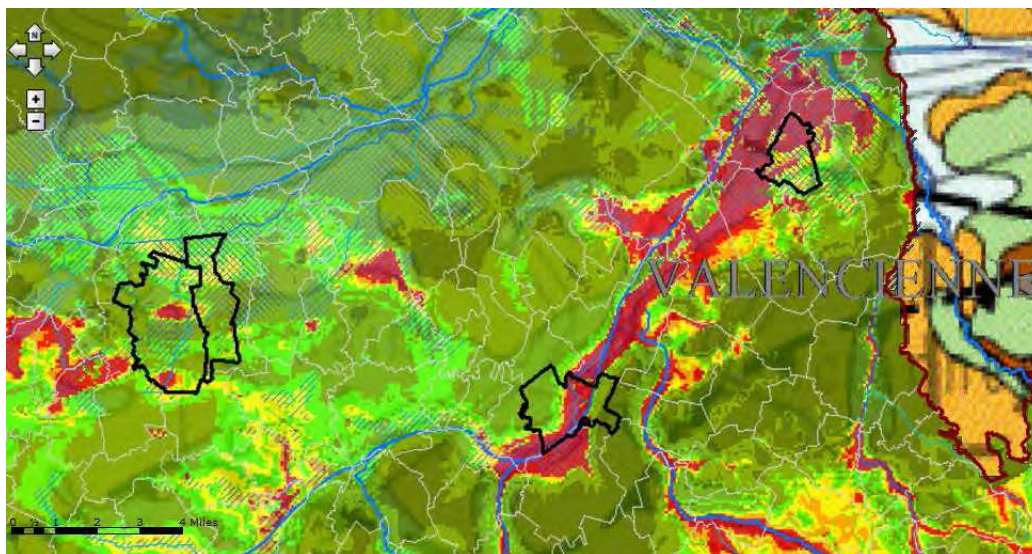
Communes de Trith-Saint-Léger, sur l'Escaut (à dr.) Somain et Fenin (à g. sur le Cavin).
