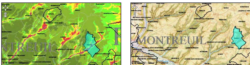
Torcy et Quilen (Pas-de-Calais, sur des affluents de la Canche, en domaine de craie)
