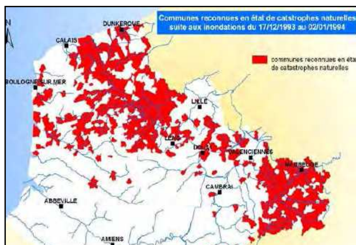
Figure 9 : Communes reconnues CAT-NAT.
