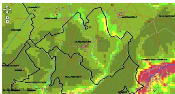
Sensibilité de la commune de Bealencourt (cartographie BRGM)
