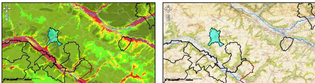
Saint Rémy-au-Bois (Pas-de-Calais, en domaine de craie)
