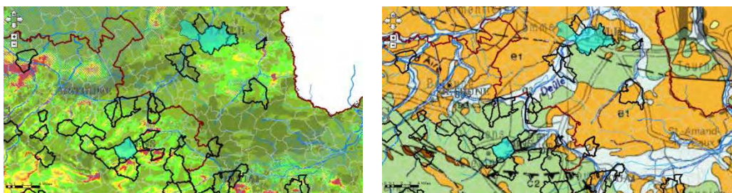
Secteur de Lens à Lille, en territoire de craie surmontée de Tertiaire
