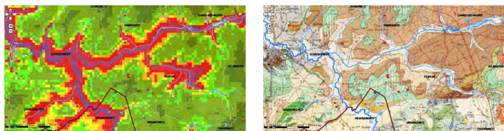
Secteur de Feron – apparition des terrains de craie
