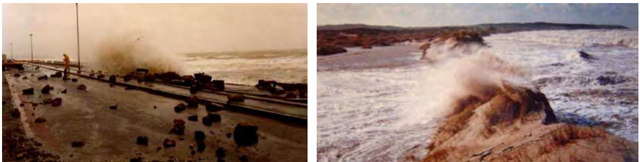
Figure 4 : Autres impacts causés par les submersions marines de fin février 1990. A gauche, perré d'Ambleteuse endommagé. A droite, rupture du cordon dunaire à Wissant. [Source : Détermination de l'alea de submersion marine intégrant les conséquences du changement climatique en région Nord – Pas-de-Calais]
