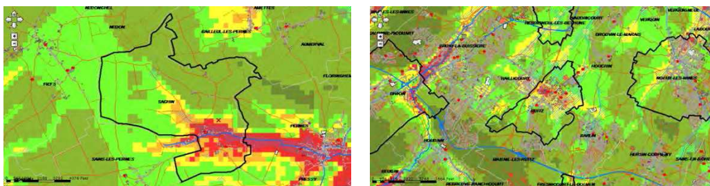
Sensibilité des communes de Sachin (à g.) et de Ruitz (à droite)
