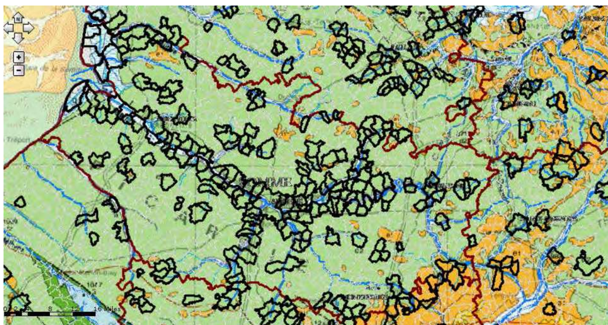
Géologie du département de la Somme, montrant l'ubiquité de l'aquifère de la craie
