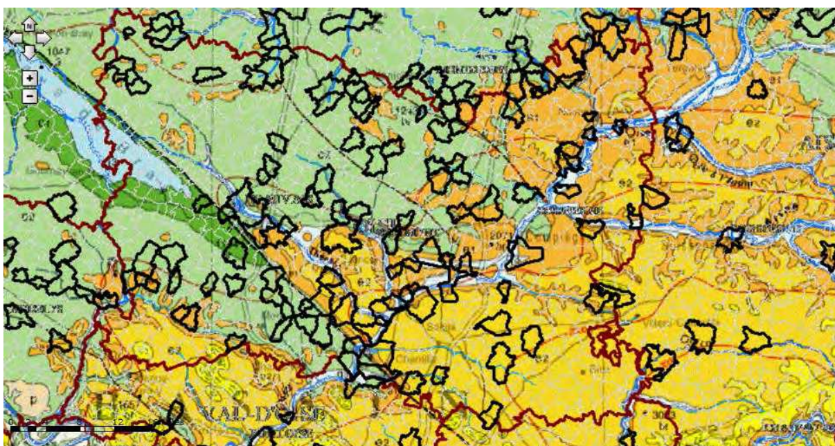
Sensibilité et géologie du département de l'Oise.
