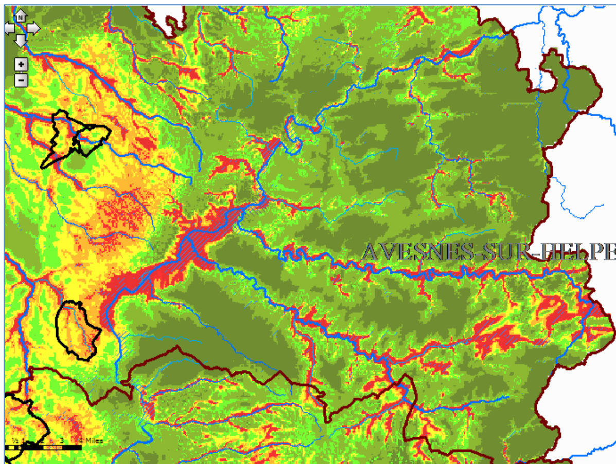
Secteur de la Sambre (cartographie de la sensibilité-version Novembre 2011-BRGM)- à gauche BAZUEL.
