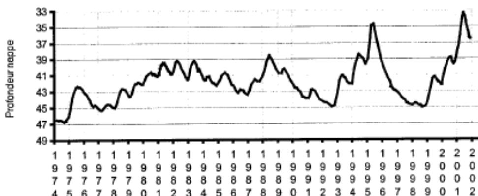
Figure 12 : Evolution piézométrique de la nappe de la craie à Huppy pour la période 1974-2002. [Source : PPRi Vallée de la Somme et ses affluents. Rapport de phase 1]
