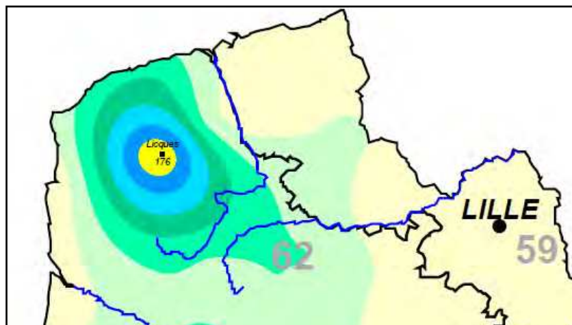
Figure 15 : Précipitations enregistrées du 12/08/06 à 6h UTC au 14/08/06 à 6h UTC. [Source : http://pluiesextremes.meteo.fr , édité le 09/08/2011]
