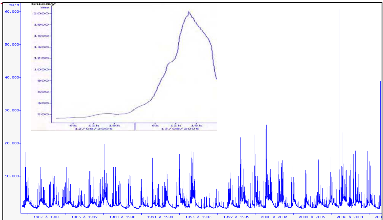
Figure 16 : Débits de la Hem enregistrés à la station de Guémy depuis 1982.
