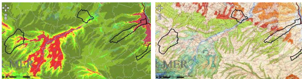
Le secteur de la craie passant sous couverture du Tertiaire (à g. la sensibilité, à dr. la géologie)
