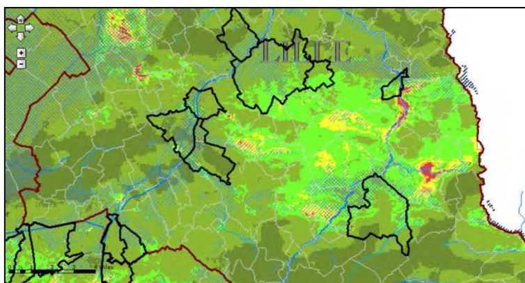
Sensibilité du secteur de Lille – cartographie BRGM Novembre 2011
