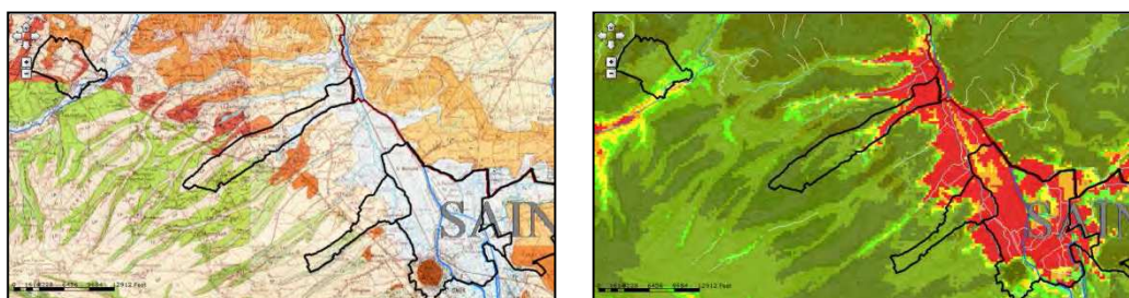
Le secteur de Saint Omer en milieu alluvial et tertiaire (à dr. la sensibilité, à g. la géologie)
