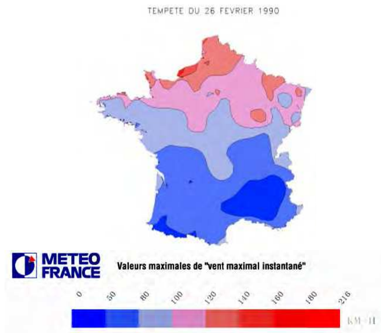
Figure 1 : Cartographie des vents maximums atteints, lors de la tempête du 26 février 1990. [Source : www.meteo.fr ]
