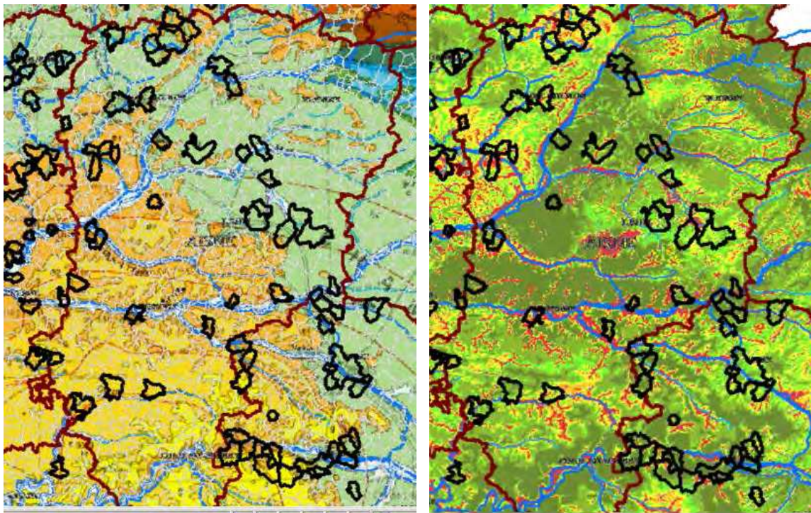
Géologie et sensibilité du département de l'Aisne
