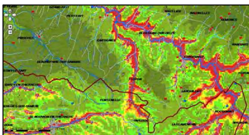
Domaine de faible sensibilité sur la commune de PRISCHE (à gauche)
