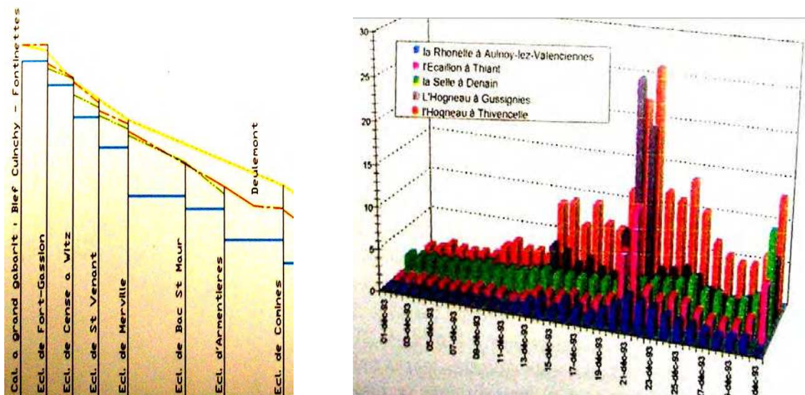
Figure 5 : A gauche, profils en long de différentes crues de la Lys.
