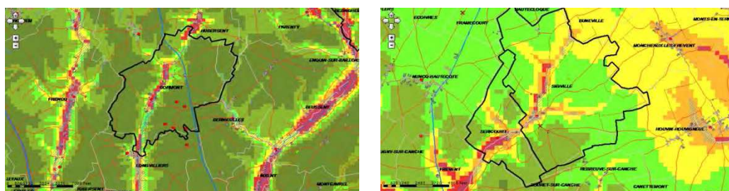
Cormont (sur la Dordogne, affluent de la Canche), Sibiville et Sericourt (bassin de la Canche)
