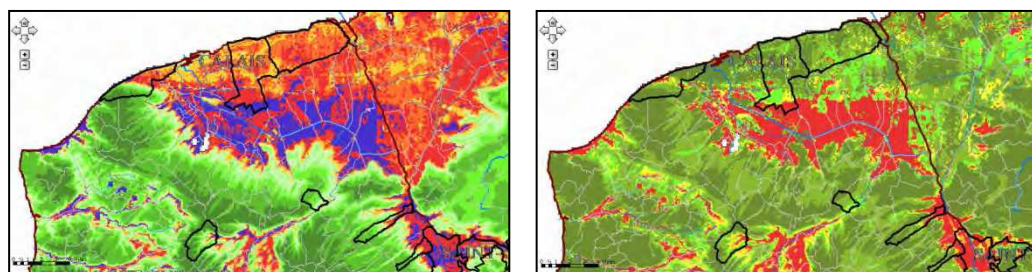
Le secteur de Calais et Dunkerque (à g. la profondeur à l'eau, à dr. la sensibilité)
