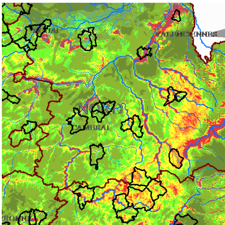
Secteur de Trith-Saint-Léger, Valenciennes, jusqu'à la frontière de l'Aisne
