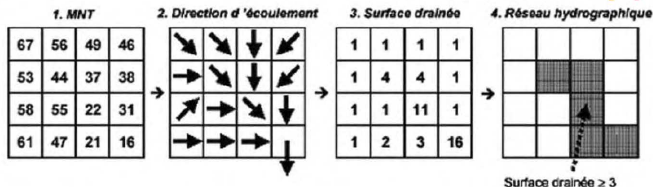
Figure 4 : Calcul du réseau hydrographique par la méthode D8 avec un seuil de surface drainée Extrait de « EXTRACTION DU RESEAU HYDROGRAPHIQUE A PARTIR DU MODELE NUMERIQUE DE TERRAIN » - Che
