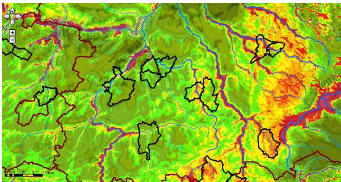
Secteur du département du Nord, zone de l'Escaut, au Nord immédiat du département de l'Aisne
