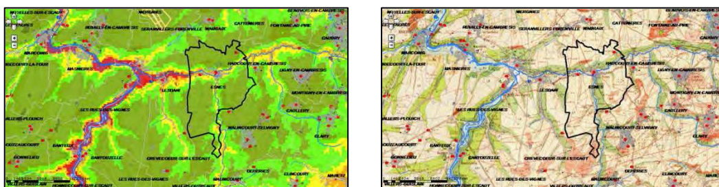
Secteur du torrent d'Esnes, en domaine de craie
