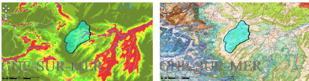
Le secteur d'Alembon (domaine de craie à l'est de la boutonnière du Boulonnais).
