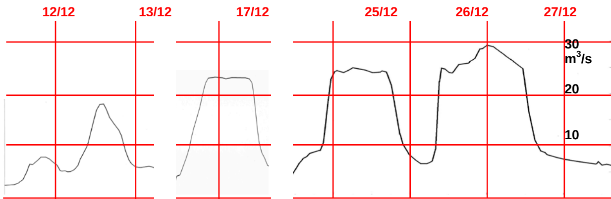
Figure 8 : Hydrogramme des 4 crues de la Lys survenues en décembre 1999 (station de Delettes), reconstitué par le CEMAGREF à partir des données sources. [Source : Rapport des crues du mois de décembre 1999]
