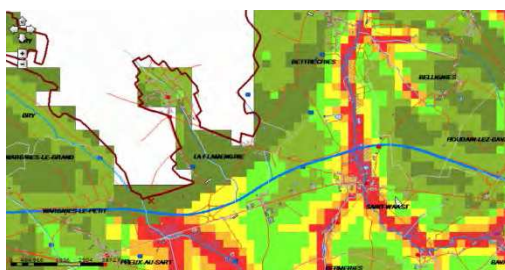
Le secteur de La Flamengrie (crétacé sous argiles à silex)
