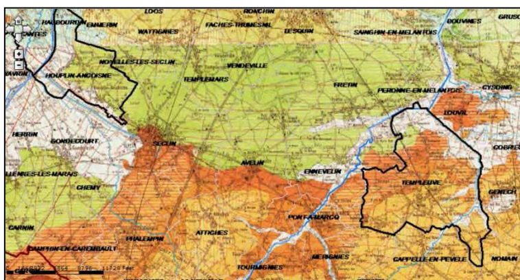
Géologie du secteur Houplin-Ancoisme
