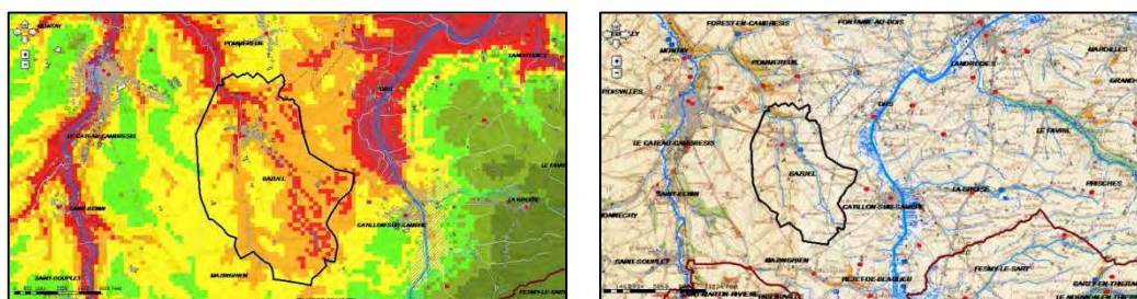
Secteur de Bazuel, à l'ouest de la Sambre
