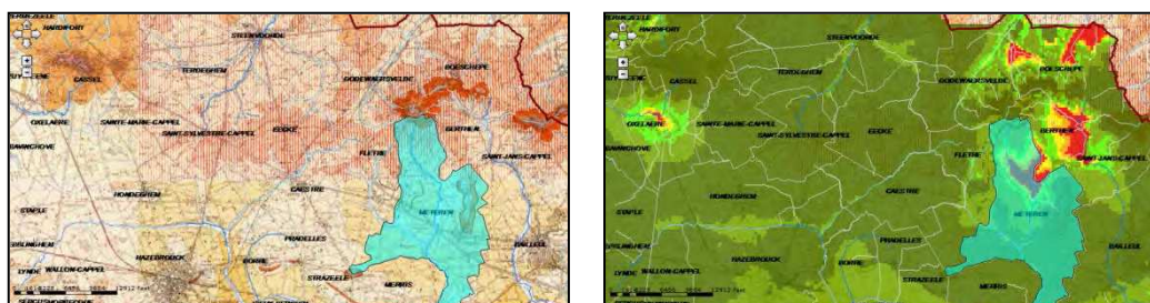
Le secteur de Meteren (à dr. la sensibilité, à g. la géologie)
