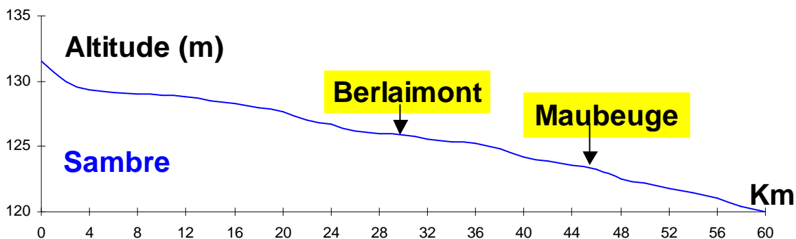
Figure 3 : Profil en long de la Sambre
