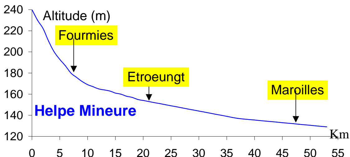
Figure 4 : Profil en long de l'Helpe Mineure
