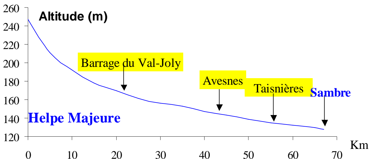
Figure 5 : Profil en long de l'Helpe Majeure
