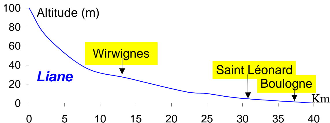
Figure 1 : Profil en long de la Liane
