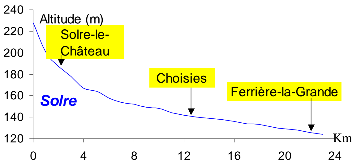
Figure 6 : Profil en long de la Solre
