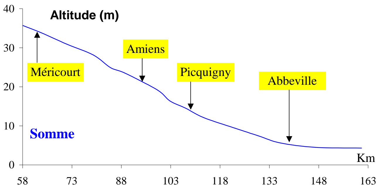
Figure 7 : Profil en long de la Somme
