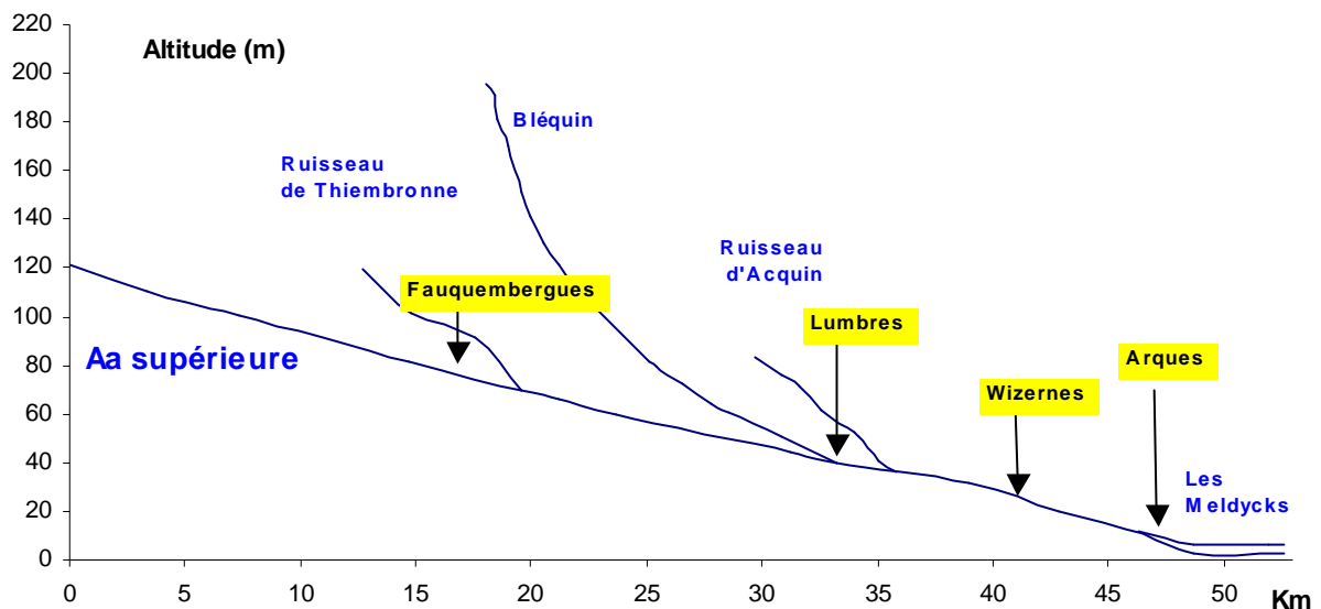
Figure 2 : Profil en long de l'Aa supérieur
